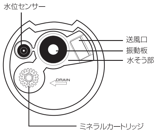
本体部
